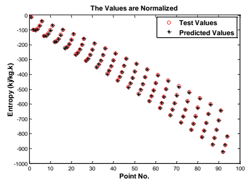
شکل (۷): ارزیابی شبکه عصبی آموزش داده شده با داده‌های نرمالیزه برای آنتروپی
