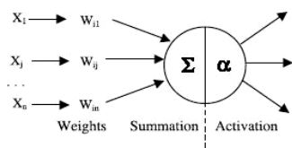
شکل (۱): پردازش اطلاعات در یک سلول شبکه عصبی
