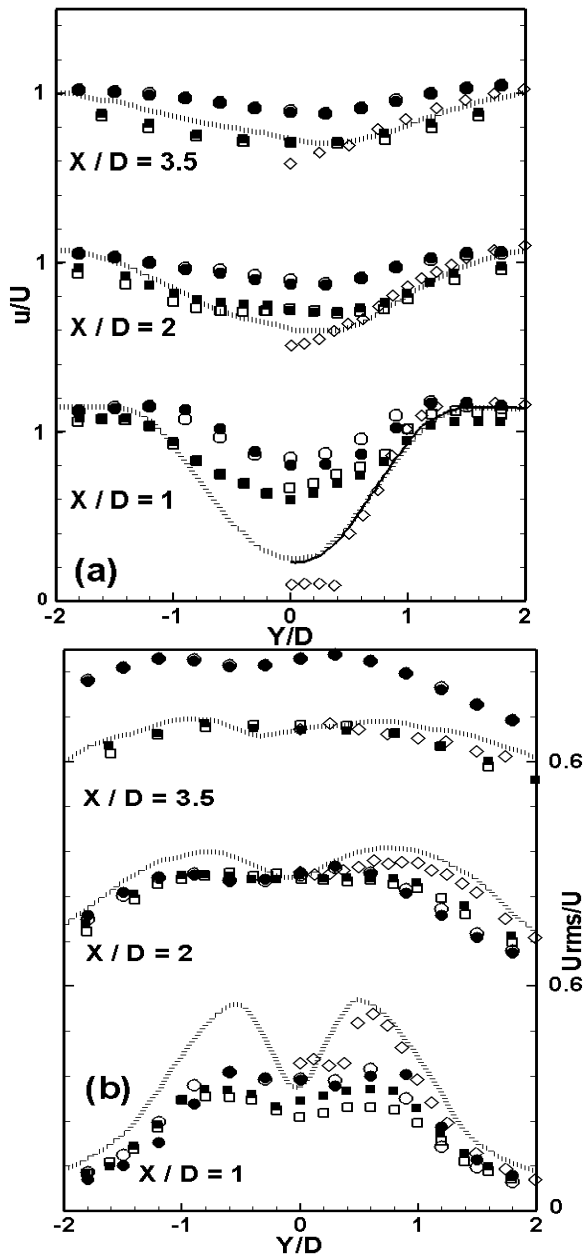
شکل (۵): نتایج توزیع سرعت (شکل a) و میزان اغتشاش‌ها (شکل b) در فاصله X/D = 1, 2, 3.5 سیلندر مربعی با زاویه حمله صفر در اعداد رینولدز 10000 و 17625 و 8700 (به ترتیب با علامت \circ و \square و \diamond ) مقایسه با نتایج تجربی ساها و همکاران [۵] (عدد رینولدز 8700 و 17625 بترتیب با علامت \square و \diamond ) و لین و همکاران [۶] (با علامت \diamond ) و عددی سوهانکار [۸] (با خط ممتد) و ونگ و همکاران [۷] (با خط چین)
