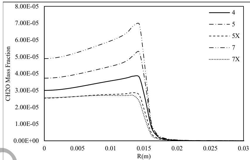
شکل ۵: اثر فیزیکی و شیمیایی تزریق دی‌اکسید کربن بر کسر جرمی فرمالدهید در فاصله ۹۰ سانتی‌متری از ابتدای مشعل
