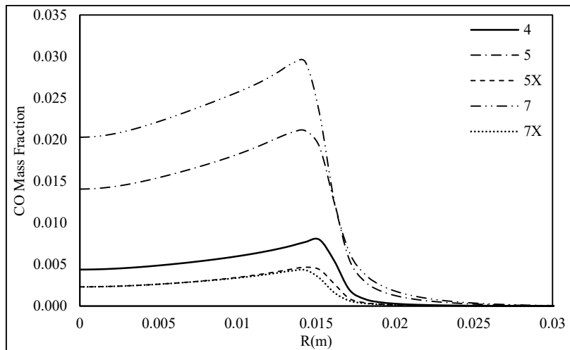
شکل ۷: اثر فیزیکی و شیمیایی تزریق دی اکسید کربن بر کسر جرمی کربن مونوکسید در فاصله ۹۰ سانتی متری از ابتدای مشعل
