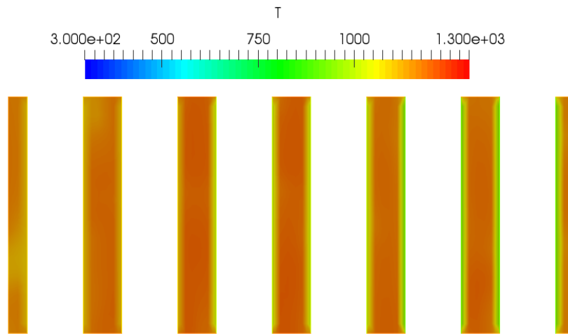
شکل ۱۶: توزیع دما در مقطع y = 0.6 (m) و 0 < x < 1.2 (m)
