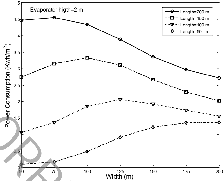
شکل ۵: اثر عرض گلخانه بر روی مصرف انرژی در ارتفاع اواپراتور ثابت برابر ۲ متر و ضریب گذردهی سقف گلخانه ۰/۶
