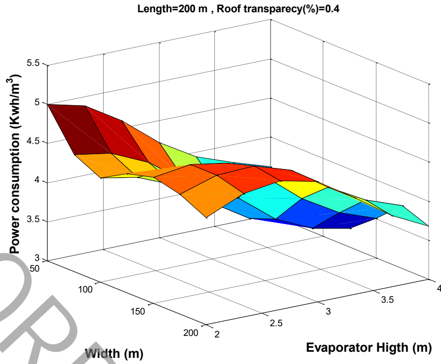
شکل ۱۱: تاثیر تغییرات عرض گلخانه و ارتفاع اواپراتور بر روی مصرف انرژی در طول گلخانه ۲۰۰ و ضریب گذردهی ۰/۴
