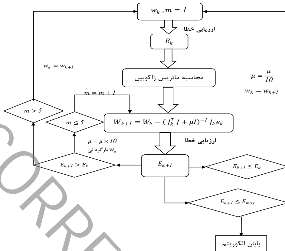
شکل ۳: دیاگرام آموزش با الگوریتم لونبرگ-مارکوآرت: w_k وزن گام جاری و w_{k+1} وزن گام بعد، E_k خطای جاری و E_{k+1} خطای گام بعد [۱۹]
