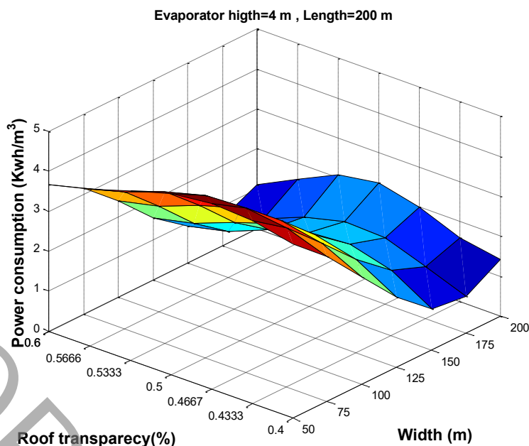
شکل ۱۰: تاثیر تغییرات عرض گلخانه و ضریب گذردهی بر روی مصرف انرژی در ارتفاع اواپراتور و طول گلخانه ثابت
