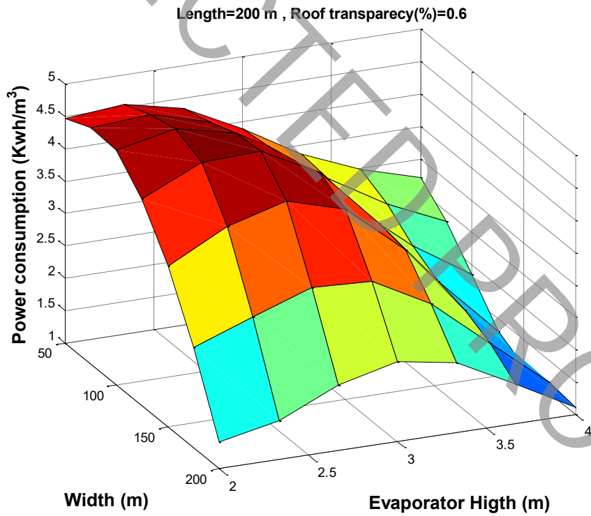
شکل ۱۲: تاثیر تغییرات عرض گلخانه و ارتفاع اواپراتور بر روی مصرف انرژی در طول گلخانه ۲۰۰ و ضریب گذردهی ۰/۶
