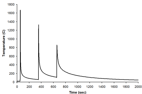
شکل (۸): چرخه حرارتی نقطه‌ای در ریشه جوش
