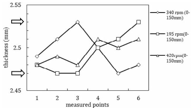
شکل ۹: مقایسه نتایج سرعت های چرخشی متفاوت سنبه با هم Fig. 9. The chart of wall thickness comparison in tested rotational speeds
