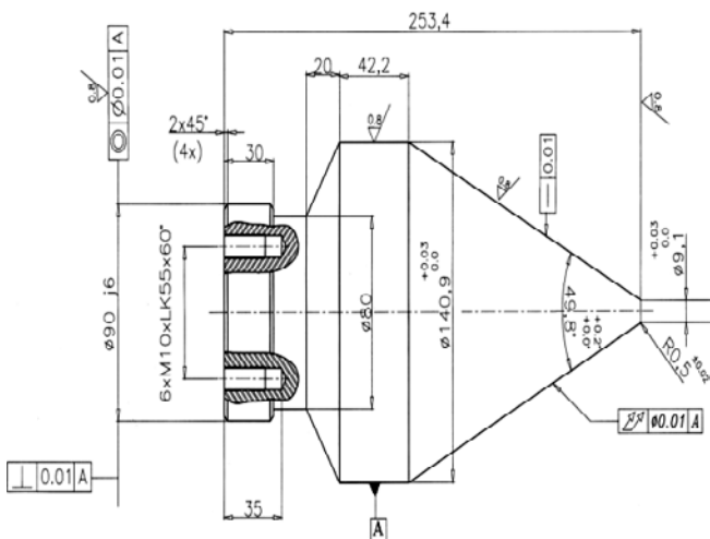
شکل ۴: مشخصات سنبه یا مندرل مورد استفاده در ساخت نمونه
