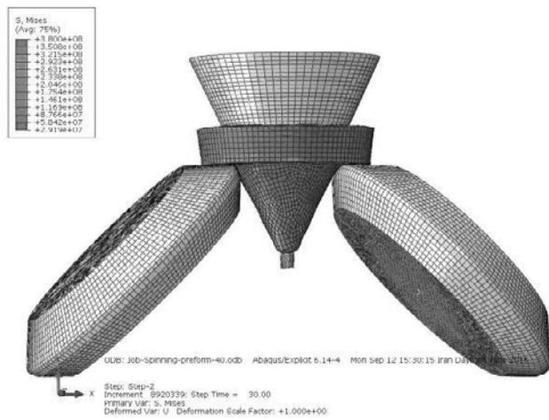
شکل ۱۳: مدل اجزای محدود فرآیند در حین تحلی بر روی پیش فرم
