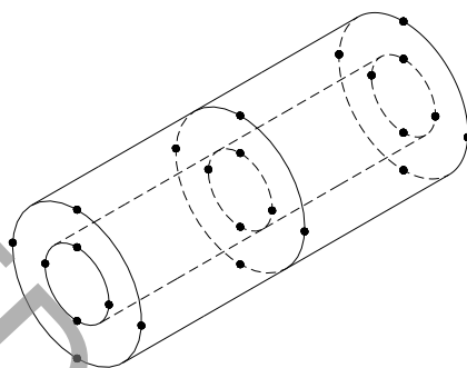
شکل ۲: مونتاژ سوپر المان به صورت سر به سر Fig.2: Superelement assembly through the axial direction
