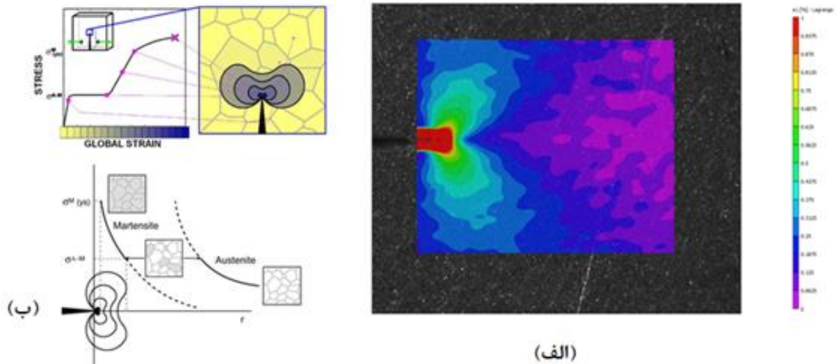
شکل ۸: (الف). الگوهای رنگی میدان کرنش در نوک ترک برای مقدار نیرویی برابر با P=120\text{ N} و نسبت طول ترک (a/w)=0.6 و (ب). میدان کرنش در نوک ترک بر اساس مطالعه رابرتسون [۱۸].
