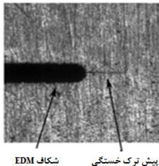
شکل ۶: ناحیه نوک ترک نمونه، متشکل از شکاف ماشین‌کاری تخلیه الکتریکی و پیش‌ترک خستگی.
