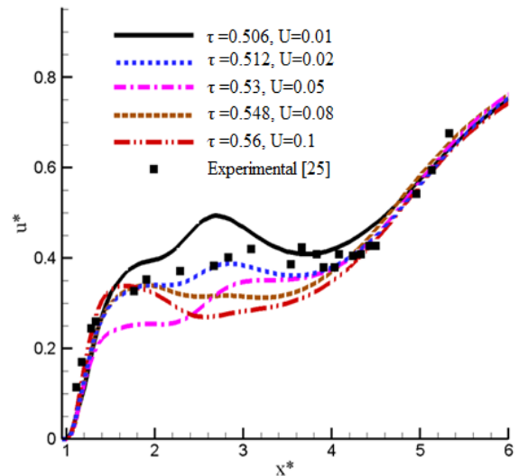
شکل ۲۵: مقایسه تغییرات مؤلفه سرعت در جهت x در پشت استوانه و روی خط افقی گذرنده از مرکز آن در زمان t^*=8 در Re=200
