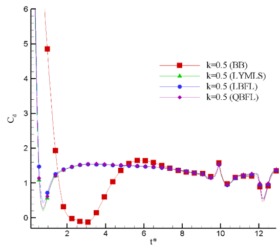
شکل ۱۵: تغییرات ضریب پسا برای استوانه دوار در شرایط k=0.5 و Re=200
