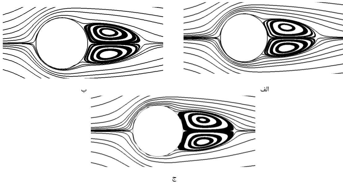
شکل ۷: خطوط جریان حول استوانه با استفاده از سه روش درون‌یابی در عدد رینولدز ۲۰: الف) روش یو خطی، ب) روش بوزیدی خطی، ج) روش بازگشت به عقب
