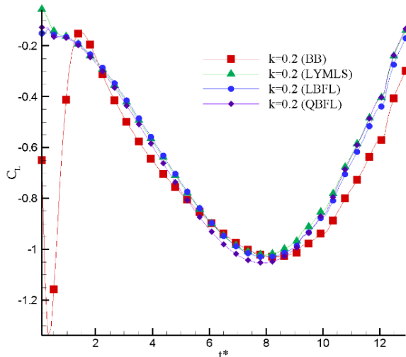
شکل ۱۴: تغییرات ضریب برآ برای استوانه دوار در شرایط k=0.2 و Re=200
