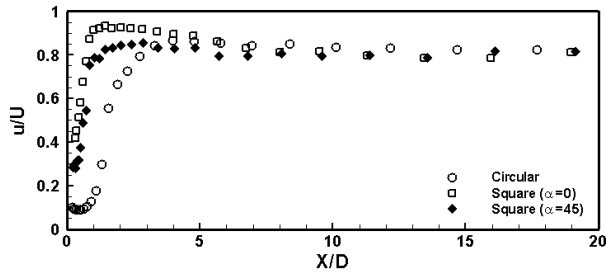
شکل (۸): توزیع سرعت بی بعد در Y/D=0 در ناحیه دنباله بر حسب طول پایین دست سیلندر مربعی با زاویه حمله صفر و ۴۵ درجه و سیلندر دایره‌ای در عدد رینولدز ۶۶۶۶
