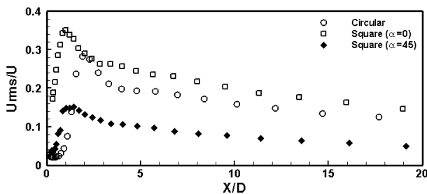
شکل (۹): توزیع شدت اغتشاشهای سرعت در Y/D=0 در ناحیه دنباله بر حسب طول پایین دست سیلندر مربعی با زاویه حمله صفر و ۴۵ درجه و سیلندر دایره‌ای در عدد رینولدز ۶۶۶۶
