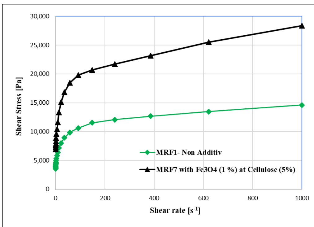
شکل ۹: مقایسه تنش برشی برحسب نرخ برش در میدان مغناطیسی 243 \text{ kA/m} و در دمای ۲۵ درجه سانتی‌گراد
