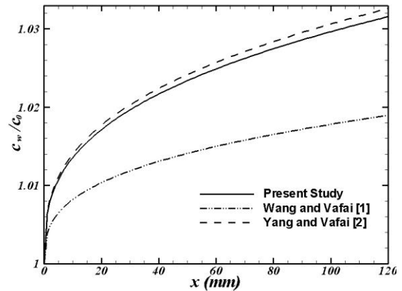
شکل ۳: مقایسه توزیع غلظت سطحی ال دی ال در امتداد محور شریان Fig. 3. Comparison of the LDL surface concentration distribution along the arterial length
