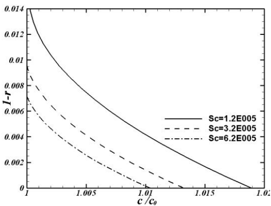
شکل ۱۳: اثر عدد اشمیت بر توزیع غلظت ال دی ال درون لایه مرزی Fig. 13. Effect of Schmidt number on the LDL concentration distribution in the boundary layer
