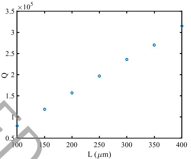
شکل ۸. تغییرات ضریب کیفیت متناظر با اولین شکل مود نسبت به طول میکروصفحه
