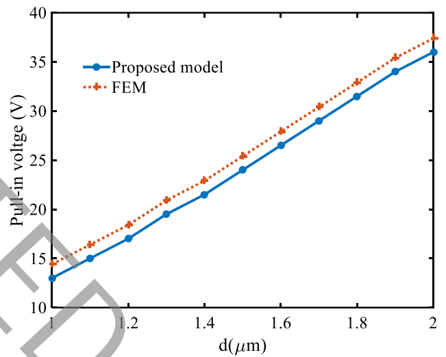
شکل ۱۲. تاثیر طول گپ بر ولتاژ ناپایداری کششی Fig. 12. The effect of gap length on the pull-in voltage
