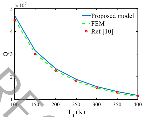
شکل ۳. تغییرات ضریب کیفیت متناظر با اولین شکل مود نسبت به دما
