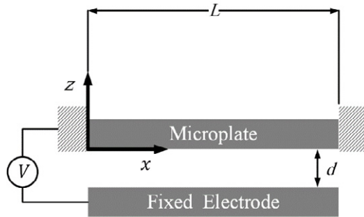
شکل ۲. شماتیک میکروصفحه تحت تحریک الکترواستاتیک Fig. 2. Schematic model of micro-plate under electrostatic actuation
