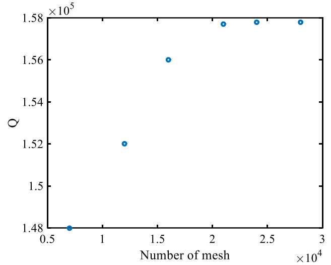
شکل ۶. تاثیر تعداد مش بر دقت محاسبه ضریب کیفیت
