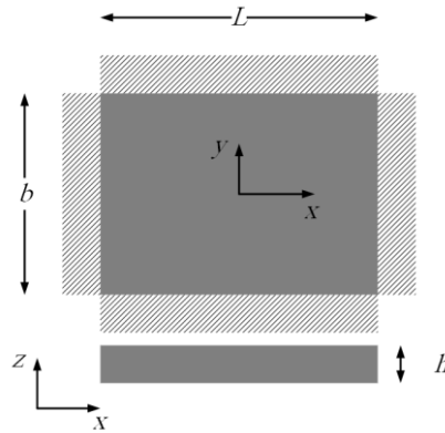
شکل ۱. شماتیک میکروصفحه مستطیلی با شرایط مرزی کاملاً درگیر
