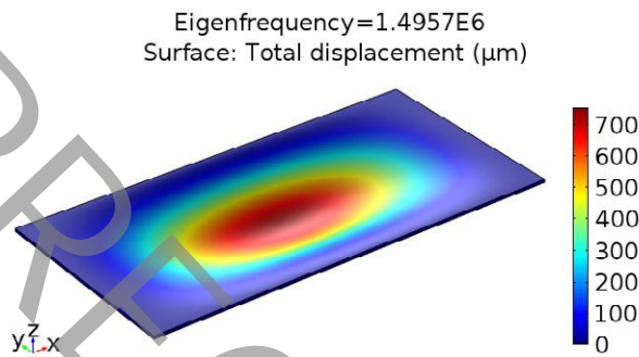
شکل ۴. اولین شکل مود میکروصفحه برای شرایط مرزی کاملا درگیر با در نظر گرفتن میرایی ترمو الاستیک
