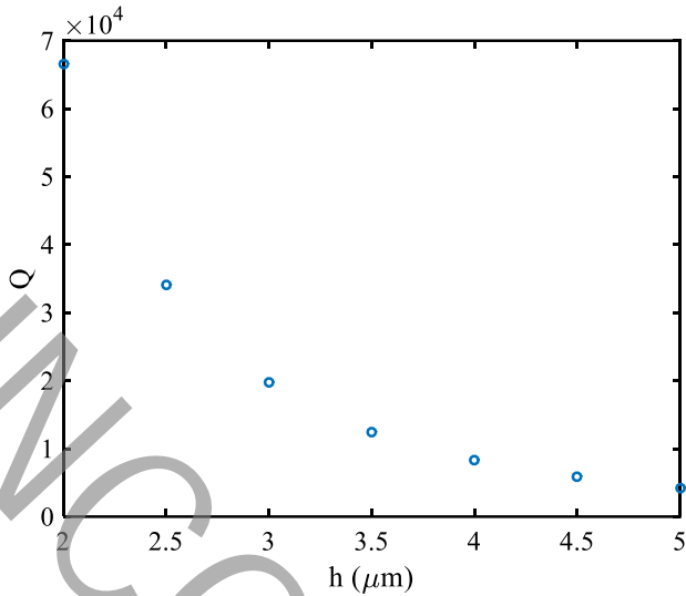
شکل ۷. تغییرات ضریب کیفیت متناظر با اولین شکل مود نسبت به ضخامت میکروصفحه
