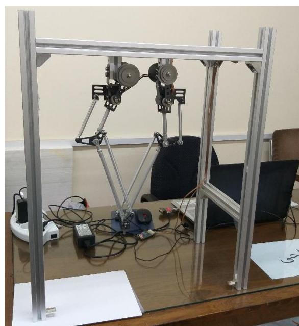
شکل ۲. ربات موازی دو درجه آزادی با دو وزنه تعادل قابل تنظیم Fig. 2. The 2-DOF parallel robot with two adjustable counterweights
