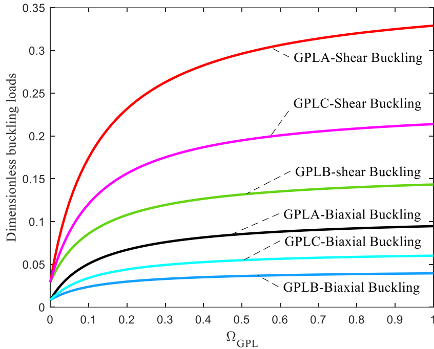
شکل ۱۶. مقایسه بار کمانش بحرانی بر حسب درصد وزنی برای ورق بیضوی تحت شرایط مرزی گیردار به ازای توزیع تخلخل نوع سوم
