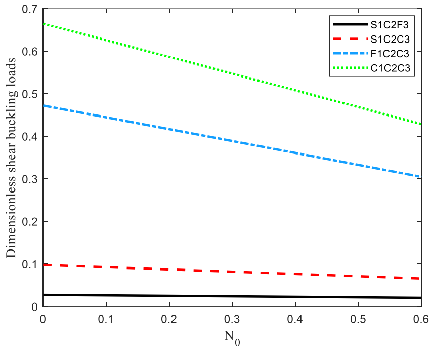
شکل ۲۳. مقایسه بار کماتش بحرانی در حالت بارگذاری برشی بر حسب ضریب پخش تخلخل برای ورق مثلثی متساوی الساقین تحت شرایط مرزی مختلف
