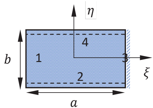
شکل ۴. ورق نانو کامپوزیتی مستطیلی تحت شرایط مرزی FIS2C3S4
