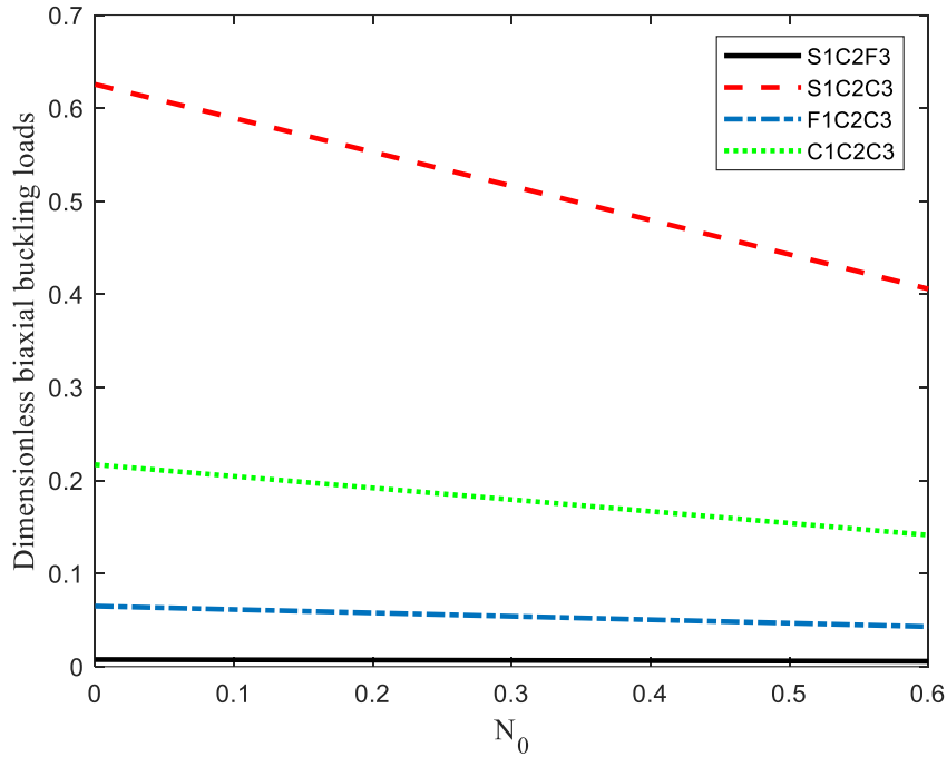
شکل ۲۲. مقایسه بار کماتش بحرانی در حالت بارگذاری دو محوری یکنواخت بر حسب ضریب پخش تخلخل برای ورق مثلثی متساوی الساقین تحت شرایط مرزی مختلف
