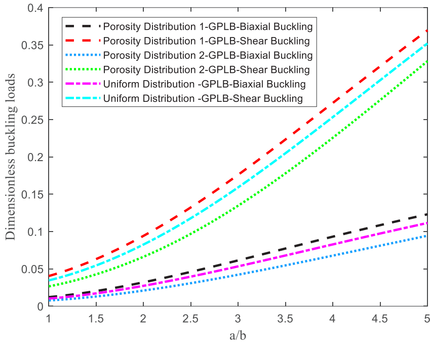
شکل ۱۸. مقایسه بار کماتش بحرانی بر حسب نسبت اقطار ورق بیضوی تحت شرایط مرزی گیردار به ازای توزیع نانو تراشه‌های گرافنی نوع دوم
