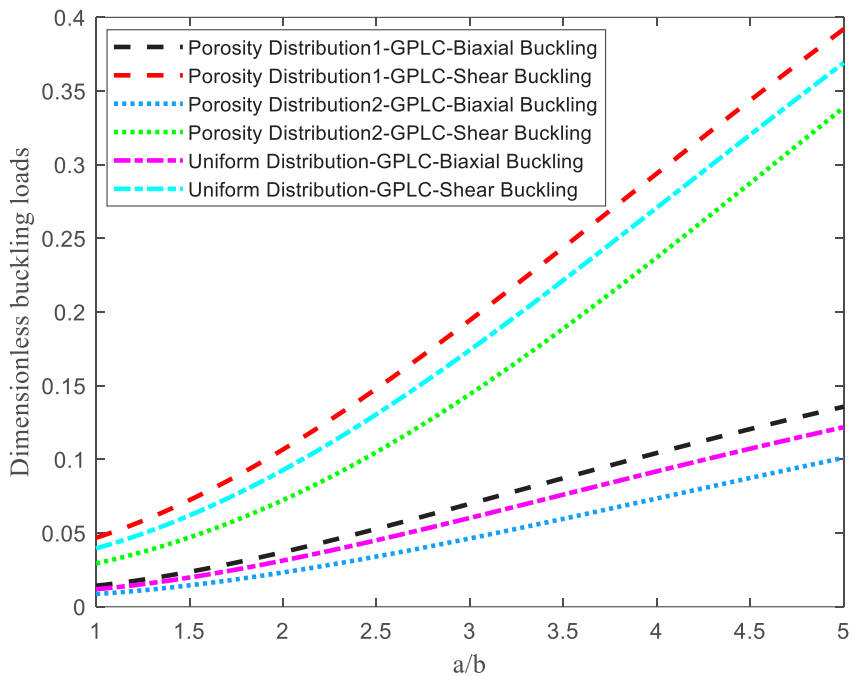
شکل ۱۹. مقایسه بار کماتش بحرانی بر حسب نسبت اقطار ورق بیضوی تحت شرایط مرزی گیردار به ازای توزیع نانو تراشه‌های گرافنی نوع سوم
