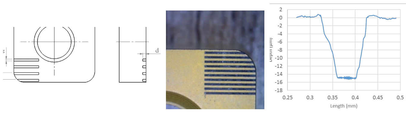
شکل ۲. تصویر میکروسکوپی سطح براده ابزارهای بافت‌دار و پروفیل سطح مقطع بافت‌ها
