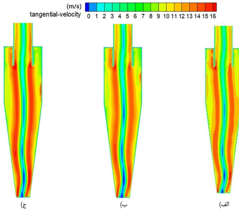
شکل ۱۴. توزیع سرعت مماسی به ازای آرایش (الف) نوع یک (ب) نوع دو (ج) نوع سه
