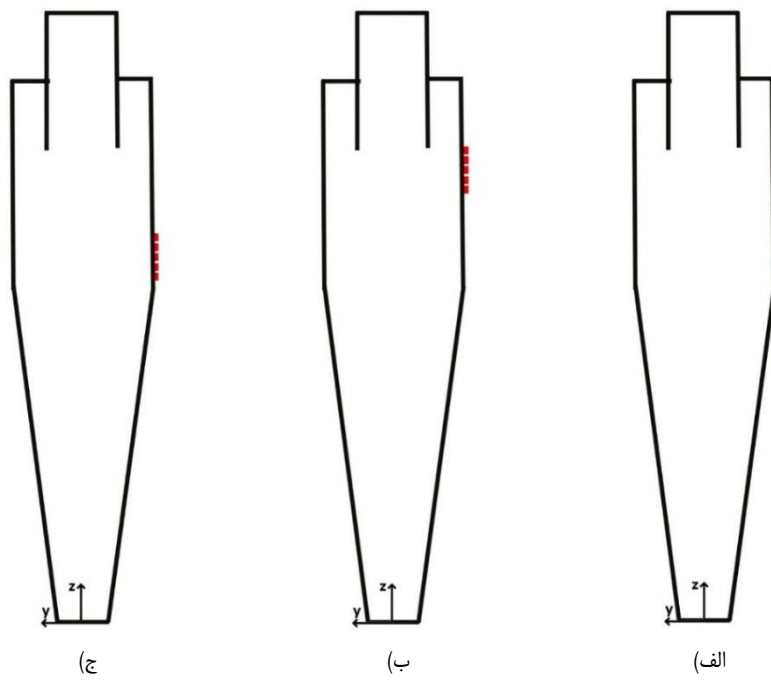
شکل ۱۳. محل نصب محرک‌های پلازما در آرایش (الف) نوع یک (ب) نوع دو (ج) نوع سه
