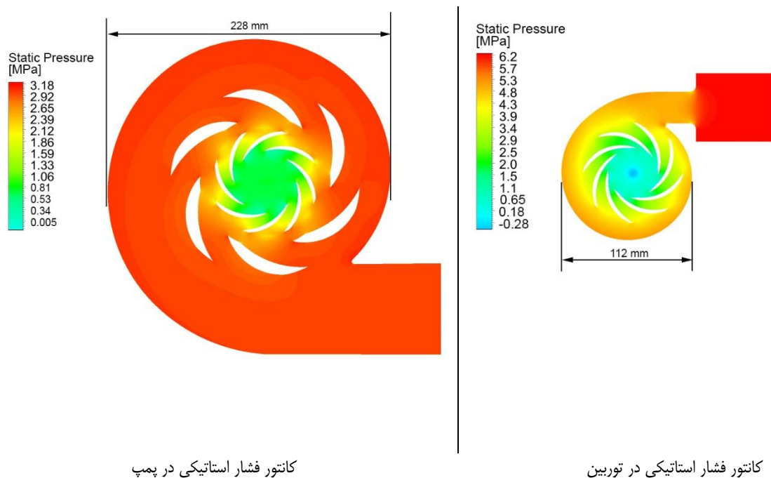
شکل ۱۱. کانتور فشار استاتیکی در دو بخش پمپ و توربین توربوشارژر
