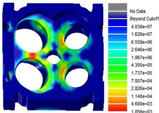
شکل ۱۳: عمر خستگی کم چرخه سرسیلندر
