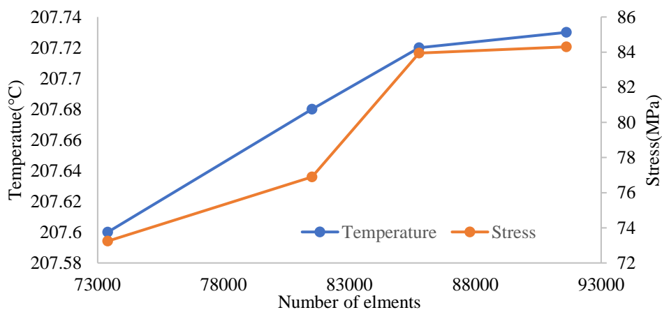
شکل ۱۲: همگرایی مش در زیرمدل سرسیلندر
