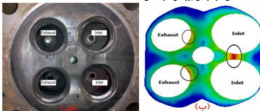
شکل ۱۷: نواحی ایجاد ترک خستگی، الف- پژوهش ژانگ و همکاران [۲۷] و ب- پژوهش حاضر
