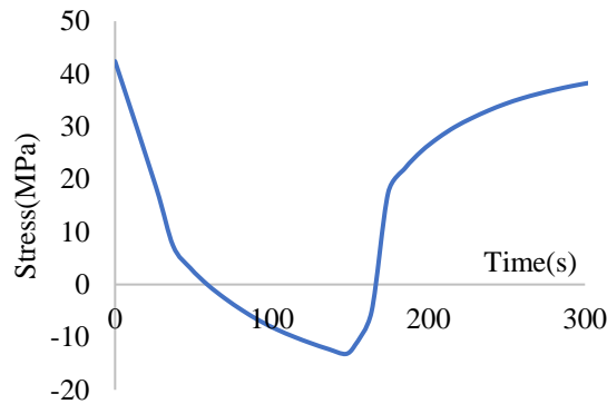
شکل ۱۱: تغییرات تنش نرمال در گره بحرانی بر حسب زمان
