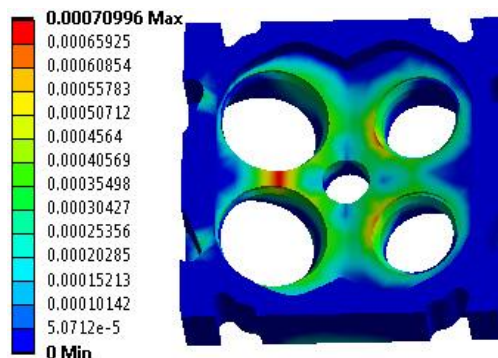
شکل ۸: توزیع کرنش پلاستیک در سرسیلندر
