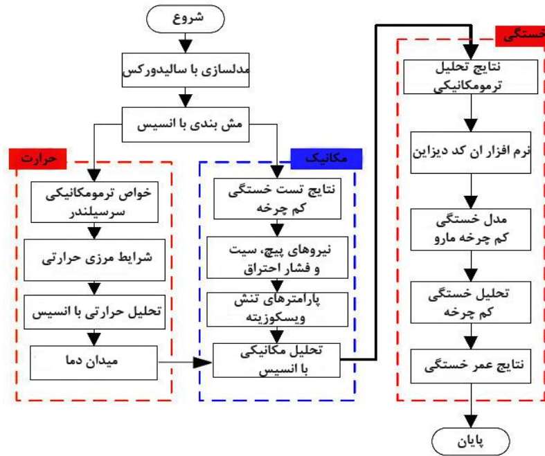
شکل ۴: فلوجارت تحلیل عمر خستگی کم چرخه سرسیلندر Fig. 4: Flowchart of the LCF analysis of cylinder head
