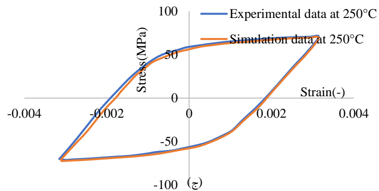
شکل ۵: نتایج تست تجربی و شبیه‌سازی شده خستگی کم‌چرخه در دمای الف - ۲۵، ب - ۲۰۰ و ج - ۲۵۰ درجه سانتیگراد
