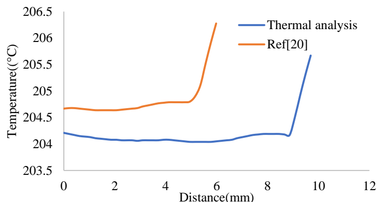
شکل ۱۶: مقایسه تغییرات دما در پل بین سوپاپ‌های دود با نتایج منبع [۲۰]
