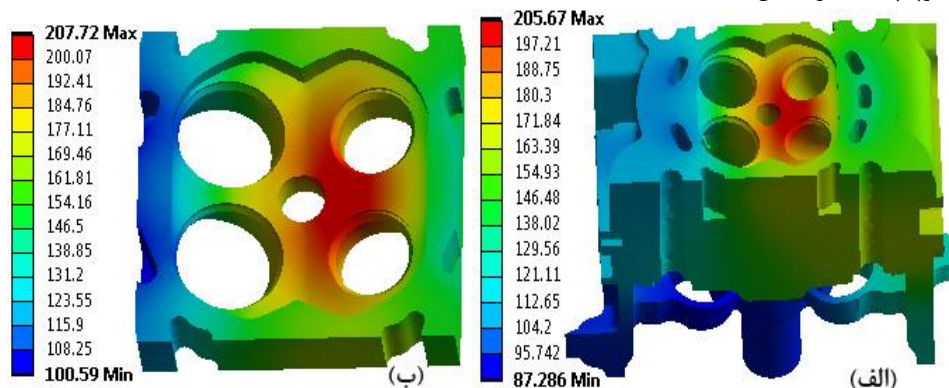
شکل ۶: توزیع دما در الف- سرسیلندر و ب- زیر مدل سرسیلندر
