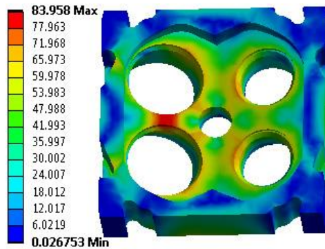
شکل ۷: توزیع تنش وان مایسس در سرسیلندر
