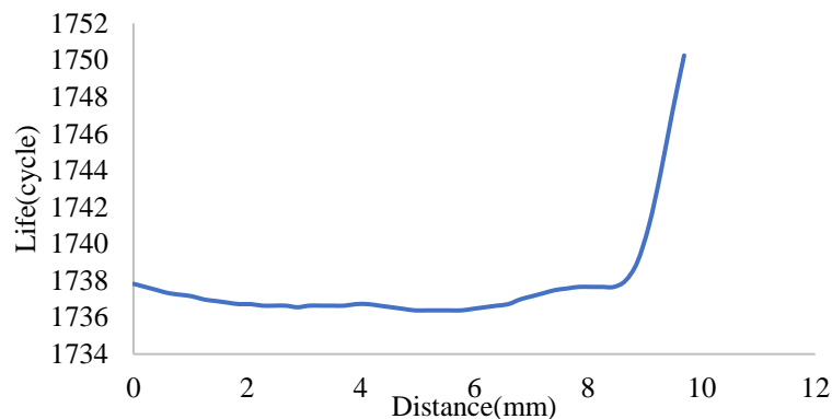
شکل ۱۵: تغییرات عمر خستگی کم چرخه در پل بین سوپاپ‌های گاز
