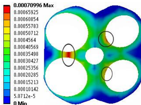
شکل ۹: نواحی بحرانی سرسیلندر
