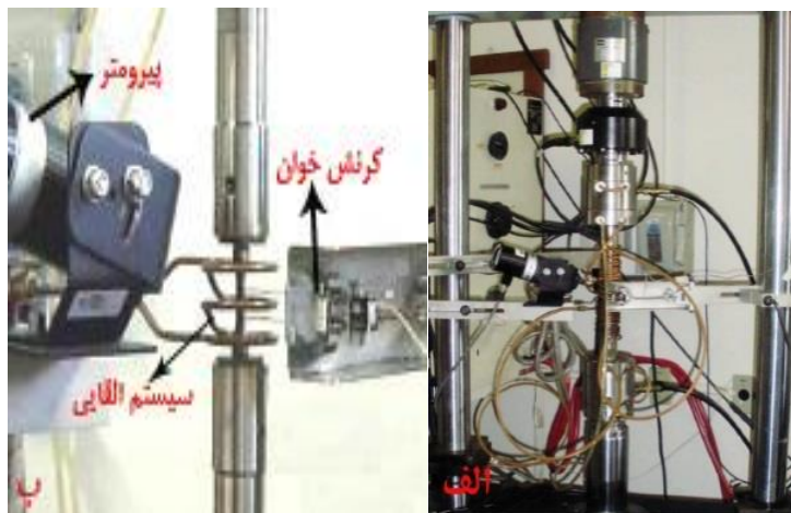
شکل ۳: الف- دستگاه تست خستگی و ب- پیرومتر، سیستم القایی و کرنش خوان
