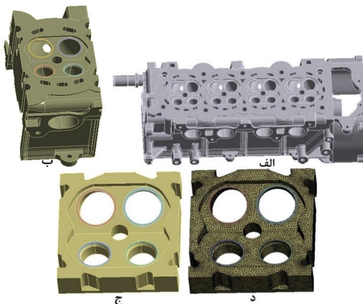
شکل ۱: الف- سرسیلندر، ب- سرسیلندر مورد استفاده در تحلیل اجزای محدود، ج- زیر مدل سرسیلندر و د- مدل اجزای محدود زیر مدل Fig. 1: (a) cylinder head, (b) cylinder head used in FEA analysis, (c) sub-model of the cylinder head and (d) finite element model of sub-model
