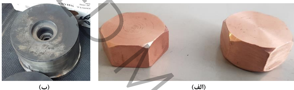
شکل ۷: الف) قطعه مسی به عنوان ابزار اسپارک، ب) شش ضلعی ایجاد شده در قالب توسط دستگاه اسپارک
