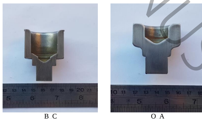
شکل ۱۴: نمای برش خورده نمونه‌ها در طول فرایند اکستروژن
