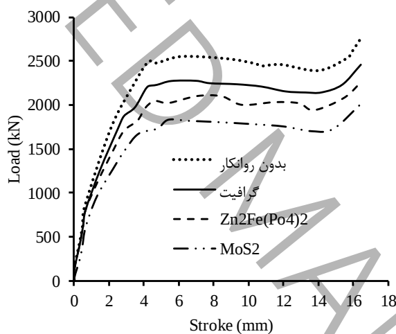
شکل ۱۵: نمودار نیرو- جابجایی در روانکارهایی با ضرایب اصطکاک مختلف در روش تجربی
