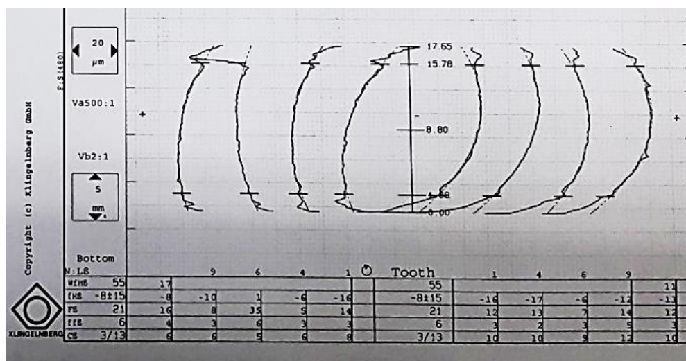
شکل ۹. نتایج آزمایشگاهی لید چرخنده ۱: الف) قبل از آزمون تجربی و ب) پس از انجام آزمون.
