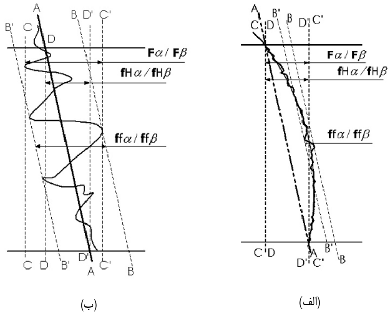
شکل ۶. مقایسه هندسه دندانه در فرآیند تولید چرخدنده با روش (الف) شیو و (ب) شاپر.
