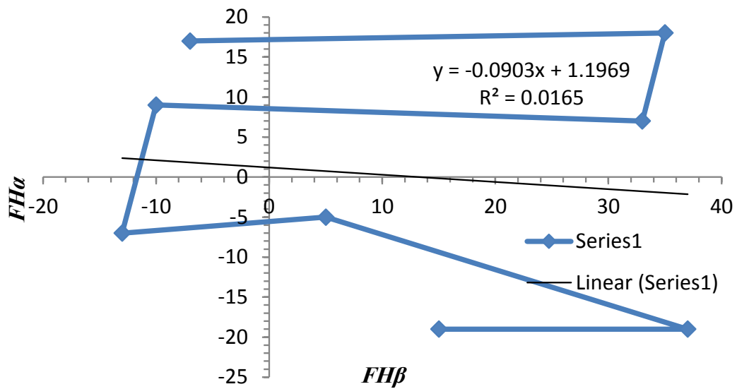
شکل ۱۲. نمودار تغییرات f_{H\alpha} - f_{H\beta} (دنده عقب).
