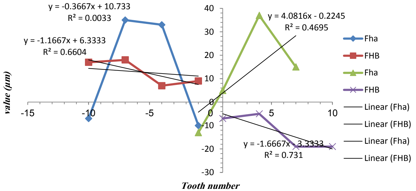
شکل ۱۱. نمودار f_{H\alpha} و f_{H\beta} بازای شماره دندانه ها در وجوه چپ و راست (دنده عقب).
