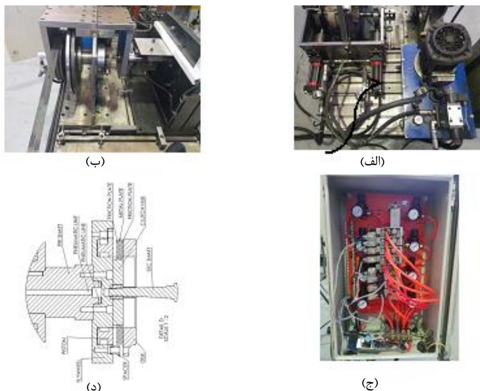
شکل ۲. مکانیزمها و اجزای بکاررفته در دستگاه آزمون استحکام پیچشی. (الف) مدار هیدرولیک دستگاه، (ب) گشتاور سنج و کلاچ چند صفحه‌ای، (ج) سیستم الکتروپنوماتیک، (د) مکانیزم کلاچ چند صفحه‌ای.
