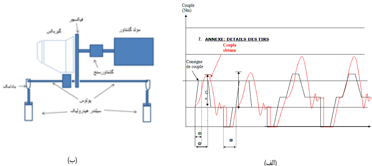
شکل ۱. (الف) نمودار اعمال بار تئوری، عملی و (ب) شماتیک عملی ارتباط اجزای سامانه آزمون جعبه دنده.
