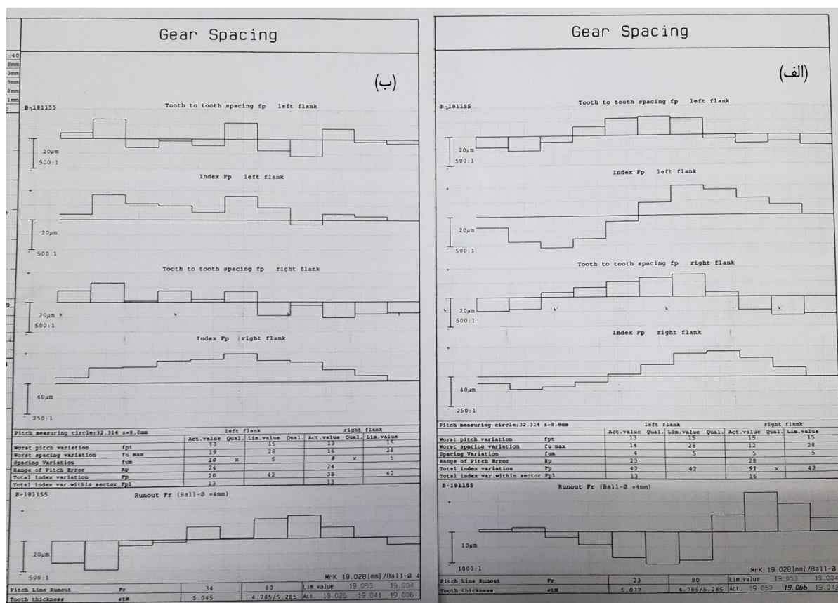
شکل ۱۰. نتایج آزمایشگاهی خطای گام انفرادی و تجمعی چرخنده ۱: (الف) قبل از آزمون تجربی و (ب) پس از انجام آزمون.
