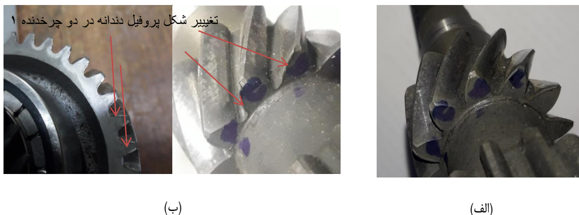
شکل ۴. (الف) پروفیل چرخ دنده قبل از بارگذاری و (ب) پس از بارگذاری پیچشی محرک و متحرک (دید از پشت چرخ دنده).
