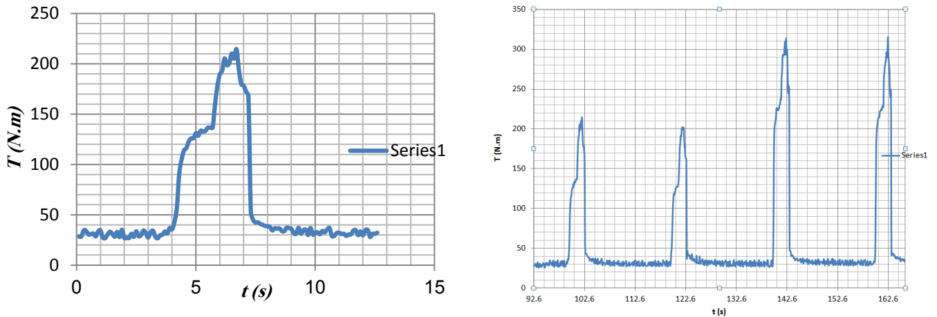
شکل ۷. (الف) نتایج آزمون انجام شده به کمک دستگاه (راست)، (ب) بزرگنمایی شده گراف با میزان گشتاور شوک ۲۰۵ نیوتن متر و ۳۱۰ نیوتن متر (چپ).
