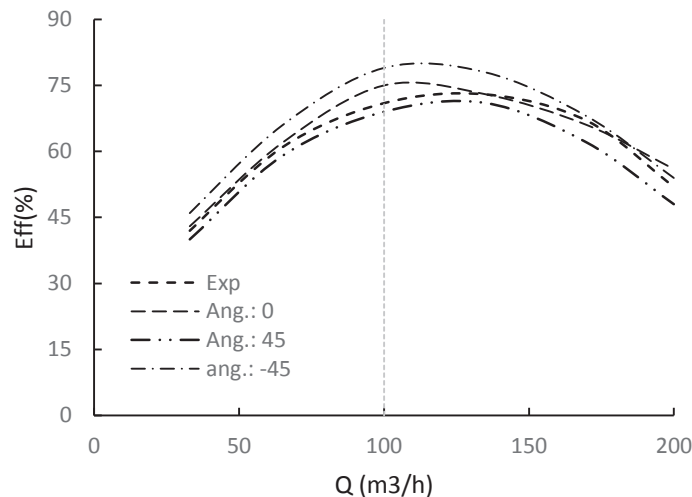
شکل ۱۰. مقایسه راندمان پمپ بدست آمده با سه زاویه ۰، ۴۵ و -۴۵ با نتایج تجربی.
