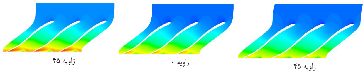
شکل ۱۲. کانتور فشار استاتیکی در پروانه در سه حالت زاویه ۴۵+ و ۴۵-.
