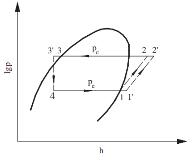
شکل ۲. دیاگرام فشار-انتالپی (P-h) سیکل پمپ حرارتی.
