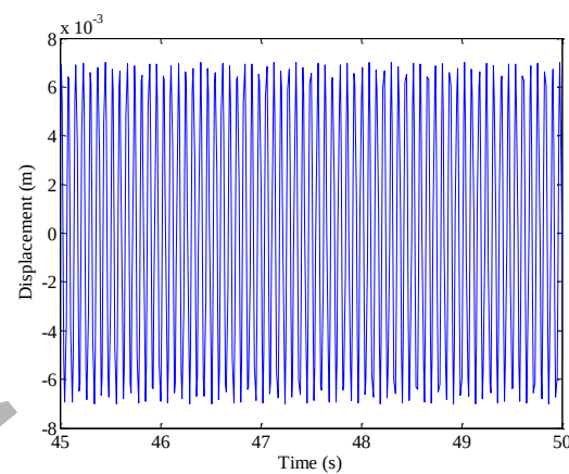
شکل ۴: تغییرات حرکت پیستون ها (الف) پیستون قدرت (ب) پیستون جابجاگر Figure 4: Piston displacement variations: a) Power piston, b) Displacer piston
