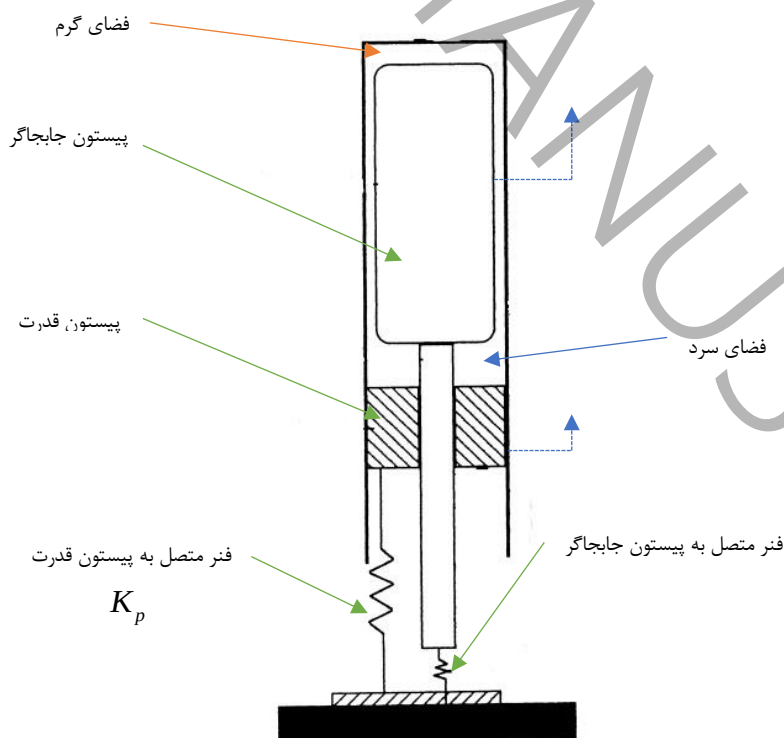
شکل ۱: موتور استرلینگ پیستون آزاد Figure 1: Free-piston Stirling engine
