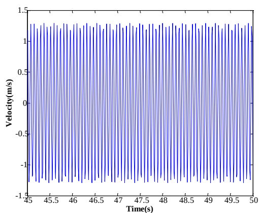
شکل ۵: تغییرات سرعت پیستون ها (الف) پیستون قدرت (ب) پیستون جابجاگر Figure 5: Piston velocity variations: a) Power piston, b) Displacer piston
