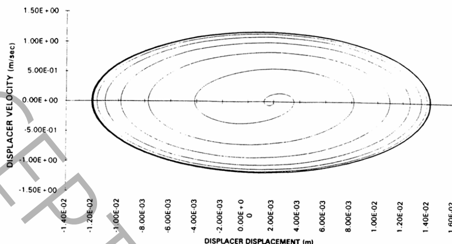
شکل ۷. نمودار فازی پیستون جابجاگر موتور B10-B [۳۸]
