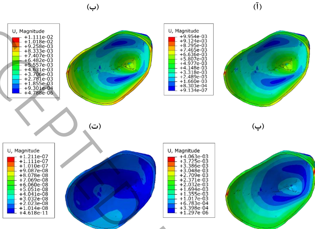
شکل ۹: توزیع جابجایی از ناحیه مجاور دندان در (PDL) با زاویه ۵ درجه (آ) ابتدای بارگذاری ( t=0.1s )، (ب) انتهای بارگذاری ( t=2.5s )، (پ) ابتدای باربرداری ( t=2.51s ) (ت) انتهای تحلیل ( t=5s )
