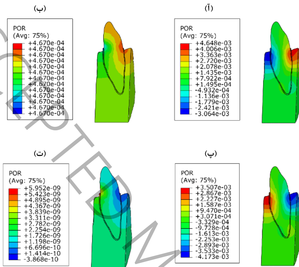
شکل ۱۲: توزیع فشار میان بافتی در (TPBC) در زمان‌های (آ) ابتدای بارگذاری ( t=0.1s )، (ب) انتهای بارگذاری ( t=2.5s )، (پ) ابتدای باربرداری ( t=2.51s ) (ت) انتهای تحلیل ( t=5s )
