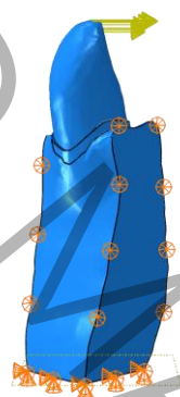
شکل ۵: شرایط مرزی و بارگذاری Fig 5: Boundary Conditions and Loading Conditions
