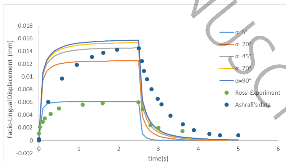
شکل ۷: نمودار جابجایی دندان برای زوایای مختلف رشته‌های کلاژن و مقایسه با نتایج راس و اشرفی
