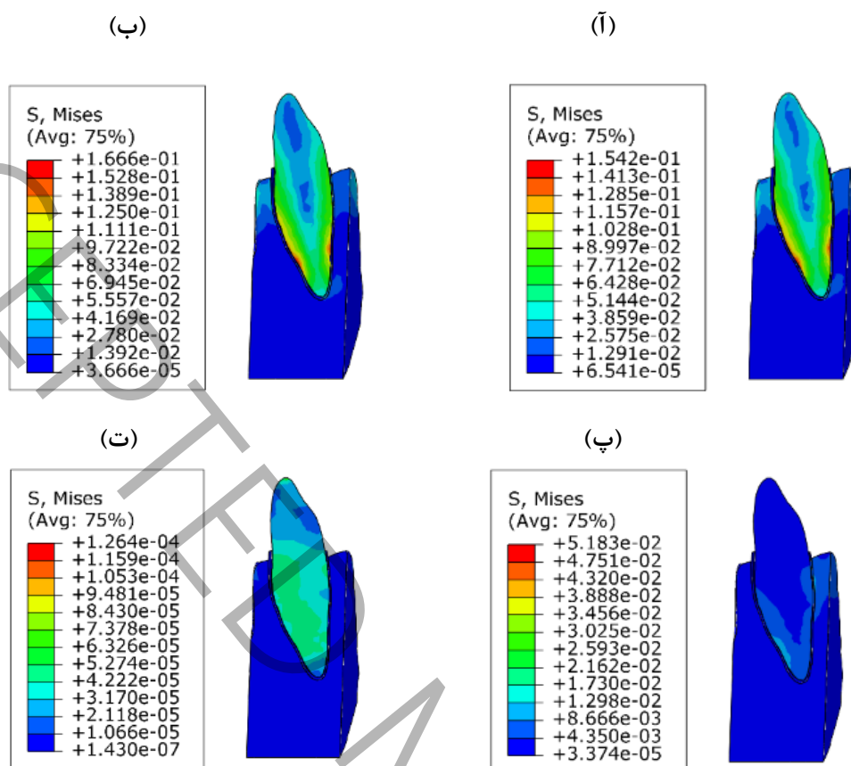
شکل ۱۳: تنش فون مایز در مقطع ساجیتال (TPBC) در زمان‌های (آ) ابتدای بارگذاری ( t=0.1s )، (ب) انتهای بارگذاری ( t=2.5s )، (پ) ابتدای باربرداری ( t=2.51s ) (ت) انتهای تحلیل ( t=5s )
