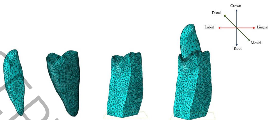
شکل ۴: سیستم پس از شبکه‌بندی Fig 4: the model after discretizing
