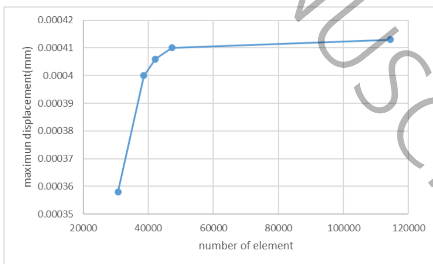
شکل ۶: تحلیل همگرایی مش برای (PDL) Fig 6: PDL Mesh Sensitivity Analysis
