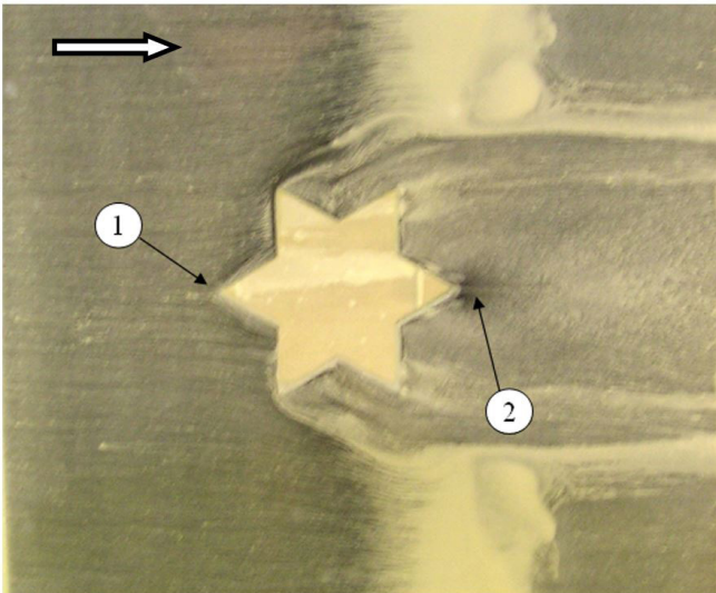
Fig. 2. Flow visualization on upper side of wing at 0° angle of attack شکل ۲: خطوط مسیر جریان از نمای بالایی بال در زاویه حمله صفر درجه
