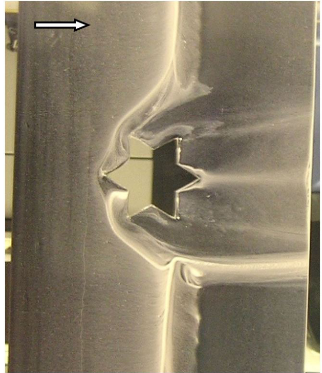
Fig. 4. Flow visualization on upper side of wing at 4° angle of attack شکل ۴: خطوط مسیر جریان از نمای بالایی بال در زاویه حمله ۴ درجه
