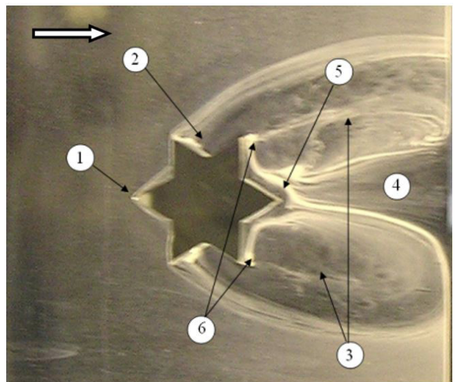
Fig. 5. Flow visualization on upper side of wing at 7° angle of attack شکل ۵: خطوط مسیر جریان از نمای بالایی بال در زاویه حمله ۷ درجه
