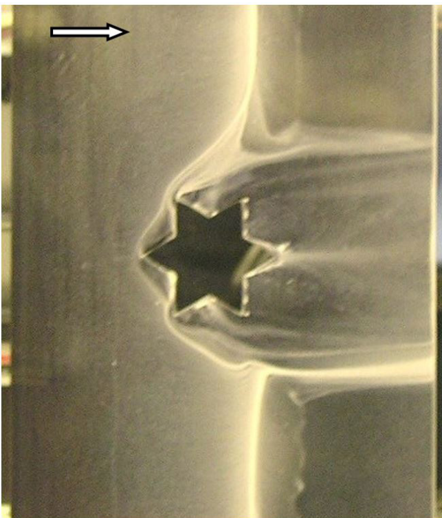
Fig. 3. Flow visualization on upper side of wing at 2° angle of attack شکل ۳: خطوط مسیر جریان از نمای بالایی بال در زاویه حمله ۲ درجه
