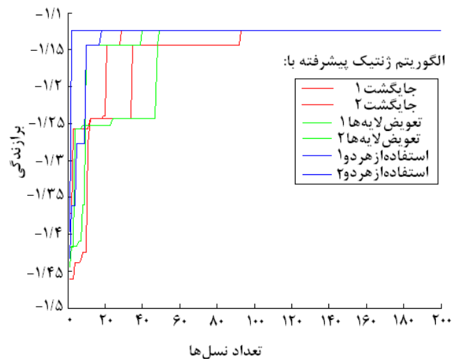
شکل (۴): نمودار برازندگی بر حسب نسل الگوریتم ژنتیک پیشرفته (a=۸۰۰mm و b=۷۰۰mm، q=۱۰KPa)
