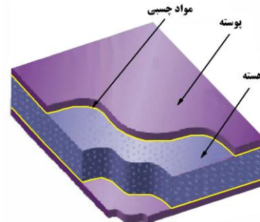
شکل (۱): نمای از یک پزل ساندویچی
