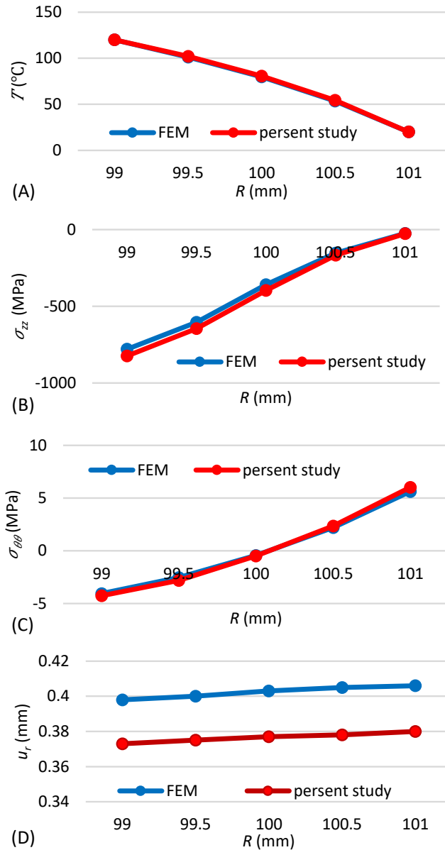
Fig. 1. Validation results; (A) thermal gradient, (B) longitudinal stress, (C) circumferential stress, (D) radial displacement
