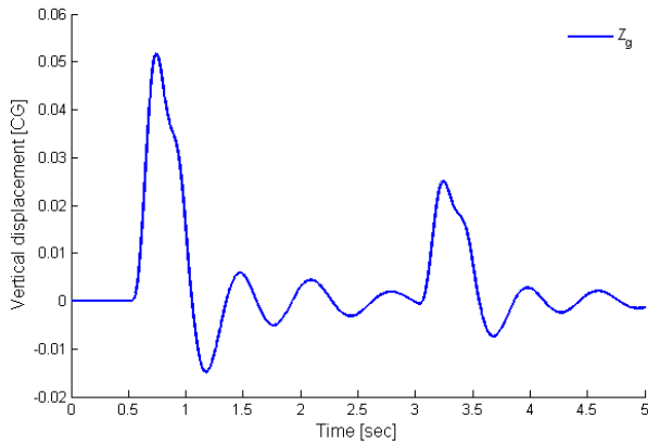
شکل ۵: سیگنال تغییر مکان عمودی مرکز جرم بدنه خودرو
