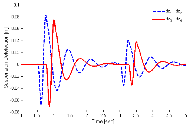
شکل ۹: سیگنال جابجایی جرم فنربندی شده
