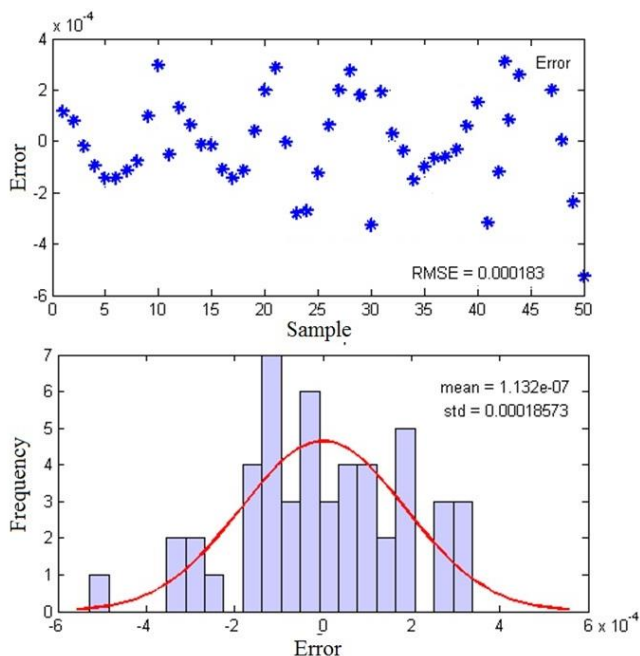
شکل ۱۲: میزان انطباق داده‌های آموزشی با مقادیر محاسبه‌شده متناظر در روش پیشنهادی تشخیص عیوب سیستم تعلیق
