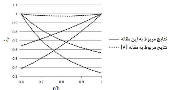
شکل ۵: مقایسه نتایج به دست آمده در این مقاله و مقاله [۸]
