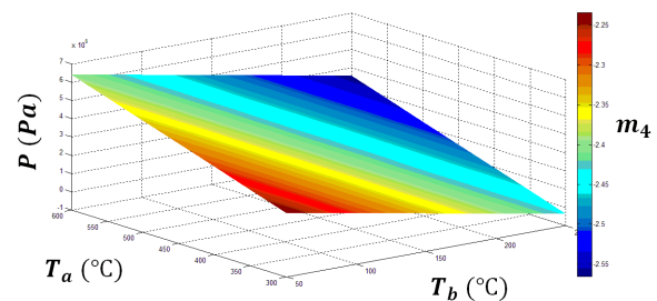
شکل ۱۲: نمودار تغییرات پارامترهای مخزن کروی با مشخصات m_1 = 3 , m_1 = 1.1 , m_1 = 3 , a/b = 0.91
