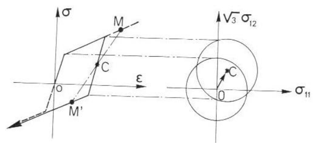
شکل ۲: آزمون کشش - پیچش تحت سختی سینماتیک و تست کشش - فشار [۱۲]
