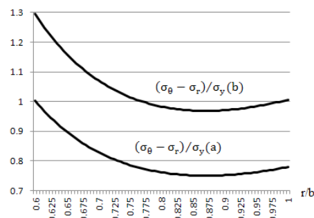
شکل ۶: تغییرات اختلاف تنش‌ها در طول ضخامت برای فشار داخلی ۴۴۴MPa و اختلاف دمای 122^\circ\text{C}
