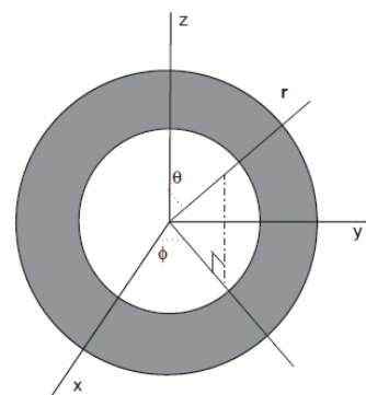
شکل ۴: مختصات کروی [۱۳]
