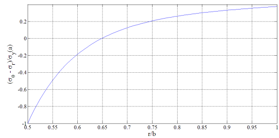
شکل ۱۰: نمودار اختلاف تنش مماسی و شعاعی (\sigma_\theta - \sigma_r) نسبت به شعاع برای m_2 = -1/1 , m_1 = 3 , b = 0/1 m, a = 0/0.5 m \Delta T = 226^\circ\text{C} , m_4 = 2 , m_3 = 3
