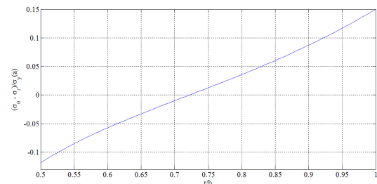
شکل ۱۱: نمودار اختلاف تنش مماسی و شعاعی (\sigma_\theta - \sigma_r) نسبت به شعاع برای m_2 = 1/5 , m_1 = 3 , b = 0/1 m, a = 0/0.5 m \Delta T = 154^\circ\text{C} , m_4 = 1/5 , m_3 = 3
